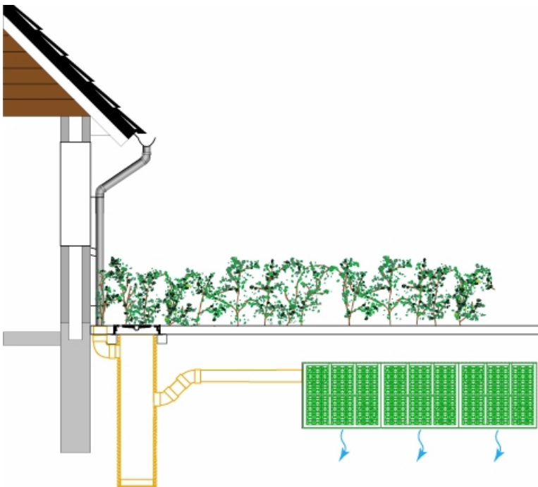
Figur 1 Opbygning af en faskine med plastkassetter
