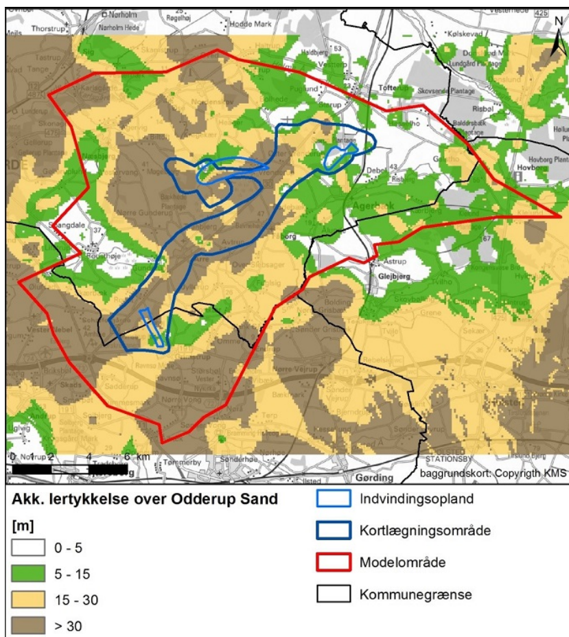
Figur 15: Akkumuleret lertykkelse over Odderup Sand/Stauning Sand
