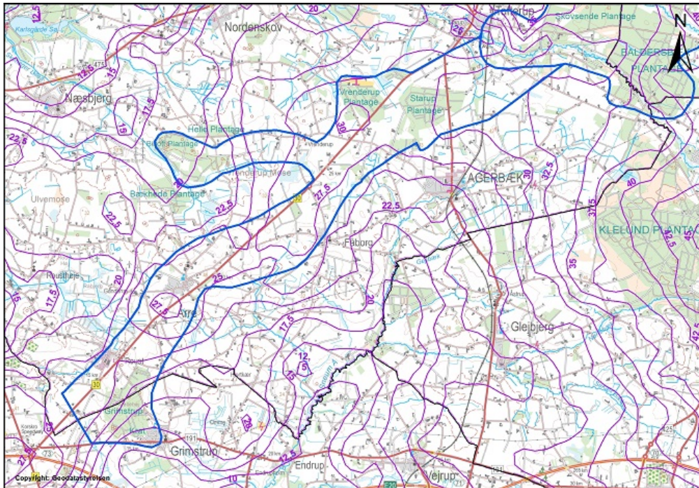
Figur 16: Grundvandspotentiale ved OSD Diagonalvejen; potentialekort fra Naturstyrelsen 2013
