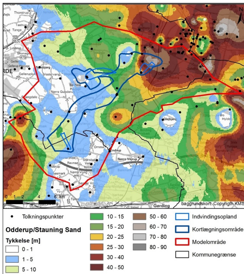
Figur 14: Udbredelse og tykkelse af Odderup Sand/Stauning Sand
