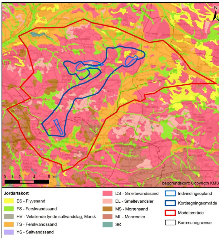
Figur 10: Jordartskort over Diagonalvejen kortlægningsområde
