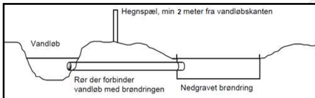
Fig 2. Principskitse for vandingssted for husdyr, udenfor vandløbsprofilen.
