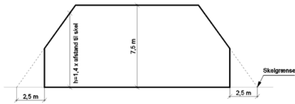
Snit, begrænsning for rumlig udnyttelse af grund.
