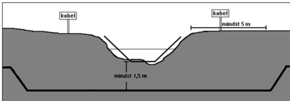
Fig. Korrekt kabelunderføring
