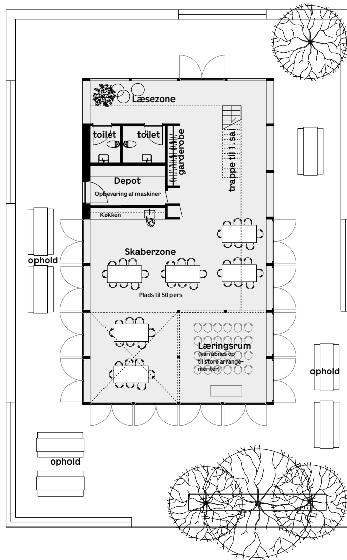
stueplan 1:200
