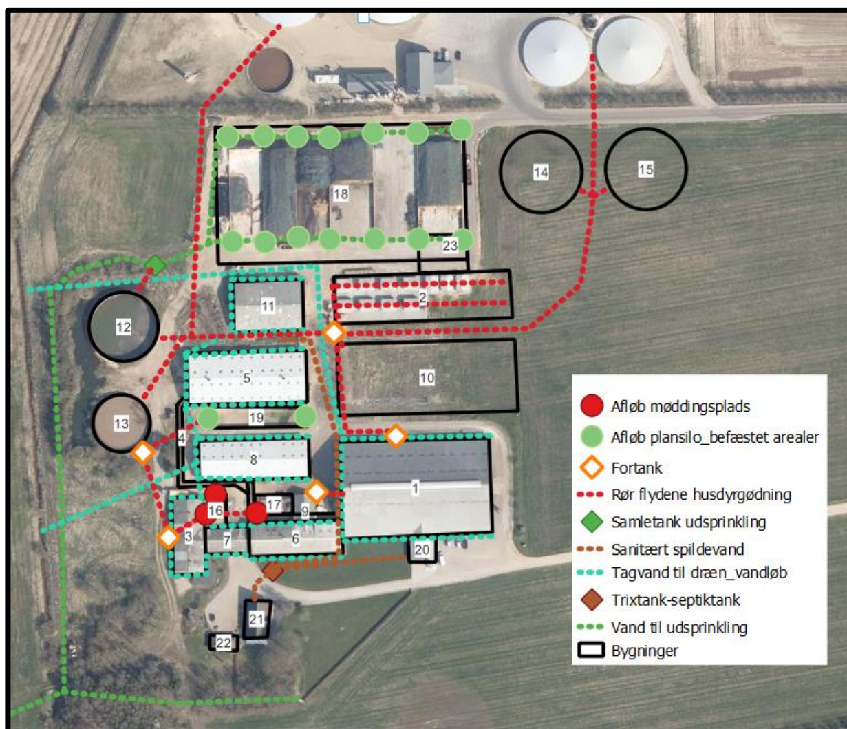
Figur 11. Afløbsplan
