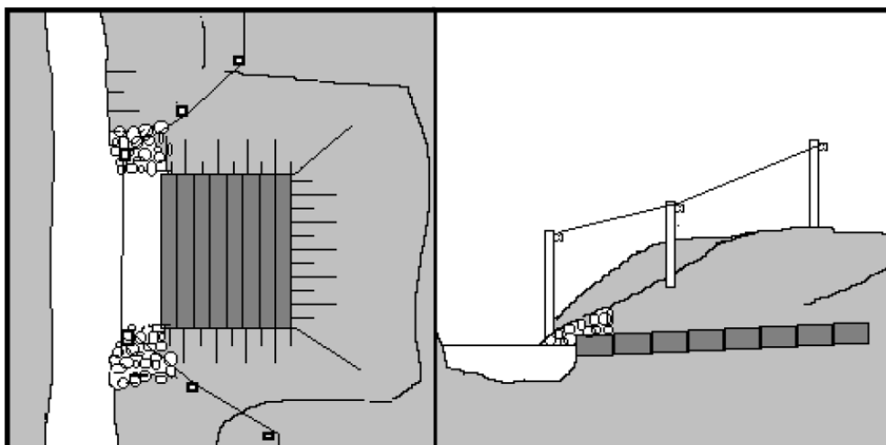
Figur 1 Principskitse for vandingssted for husdyr, indenfor vandløbsprofilen.
