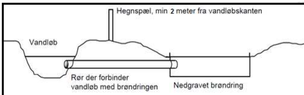
Figur 2 Principskitse for vandingssted for husdyr, udenfor vandløbsprofilen.
