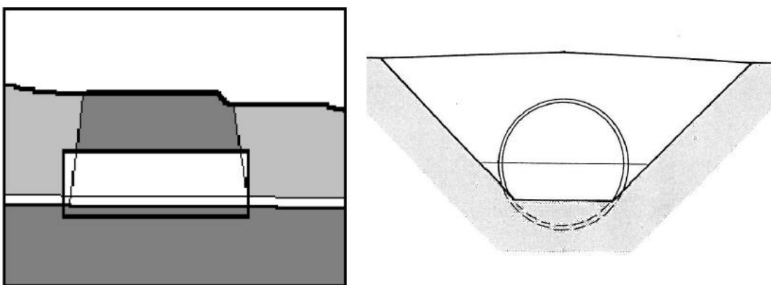
Figur 1 Længde- og tværsnit af korrekt anlagt rørbro, som er nedgravet med 1/5 del af rørdiameteren.
