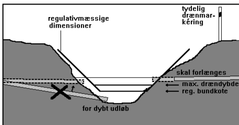
Figur 1 Forkert og korrekt anlagt drænudløb.
