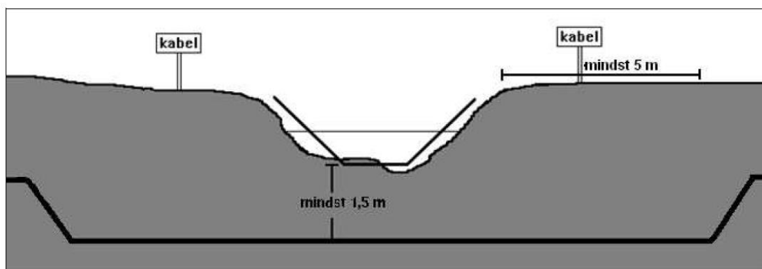
Figur 1 Korrekt kabelunderføring
