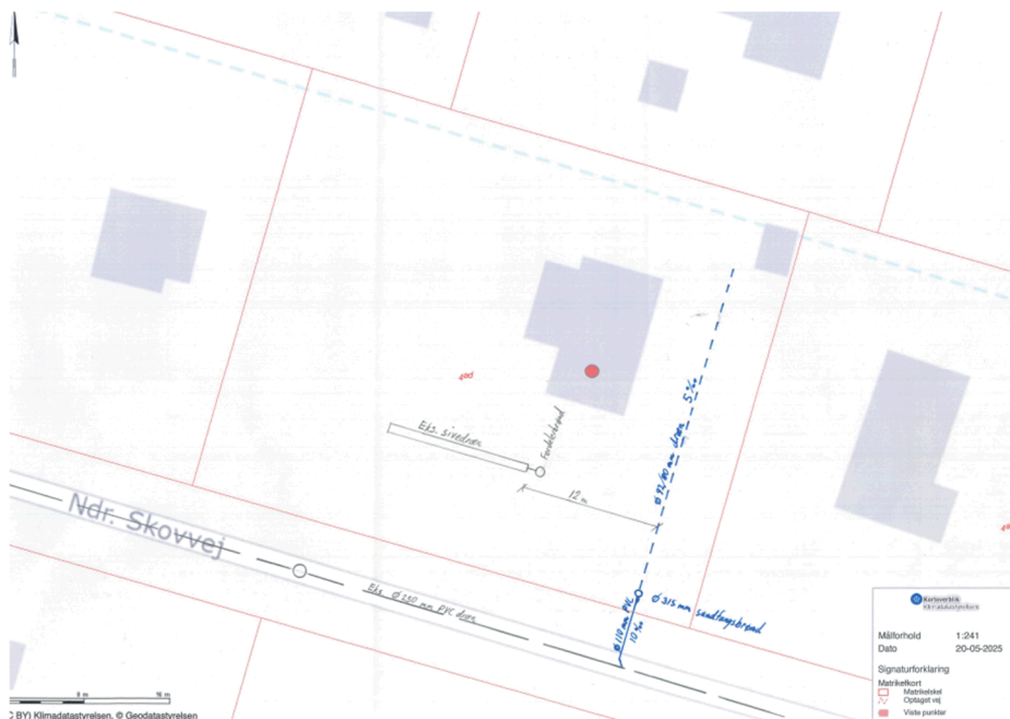
Fig. 1 Ndr. Skovvej 8 med indtegnet dræn og sandfangsbrønd, som sluttes til vandløb.
