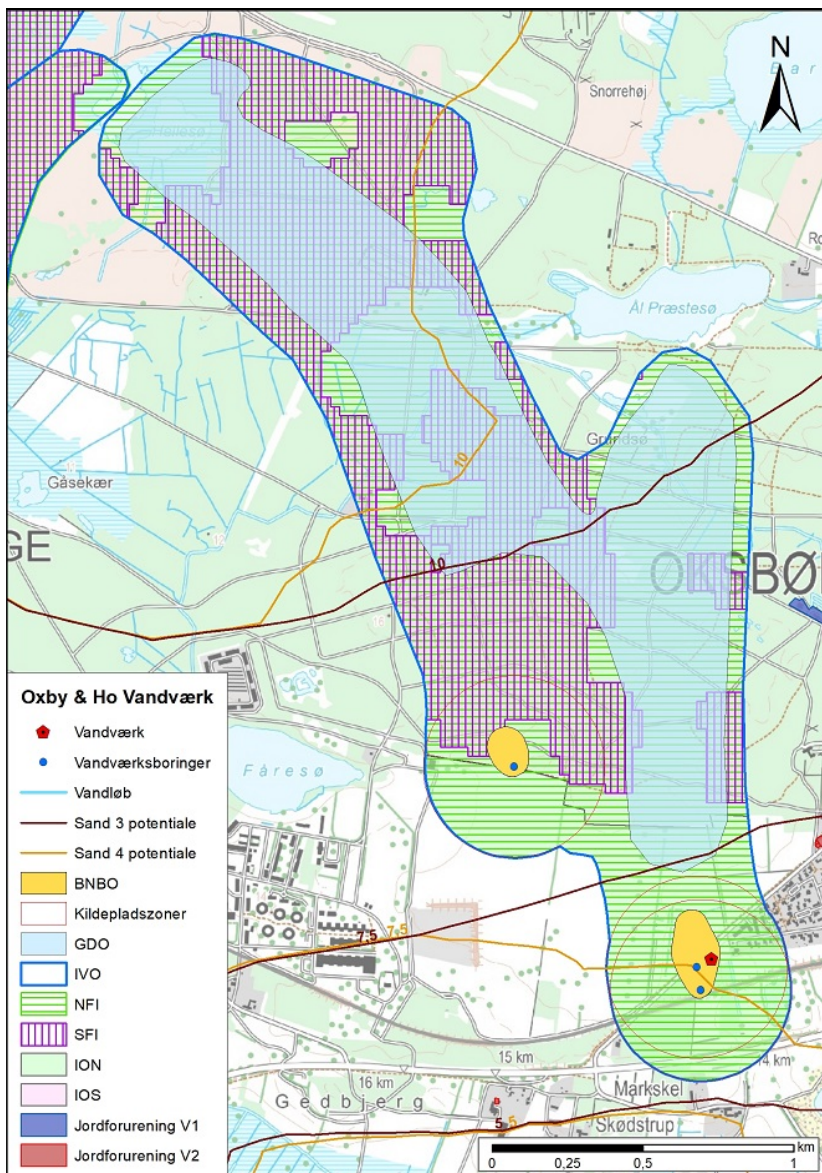
Figur 42: Oxsbøl Vandværk med IVO, GDO, NFI, SFI, ION, IOS, kildepladszonen mv. og grundvandspotentiale for vandværkets primære magasiner Sand 3 og Sand 4
