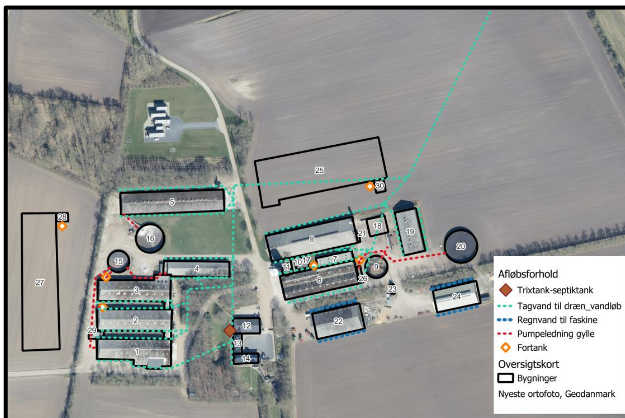
Figur 10. Afløbsplan
