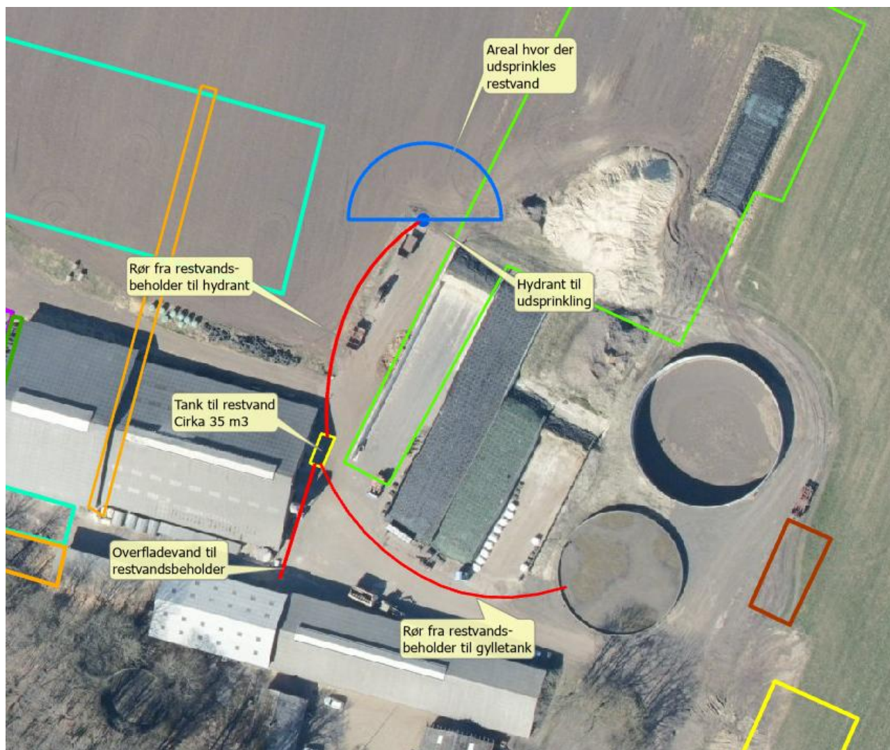
Figur 13. Rød streg viser rør med restvand og overfladevand i nudrift.
