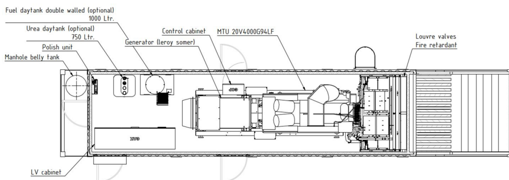
Figur 7: Eksempel på opbygning af containerløsning for nødgeneratorer.
