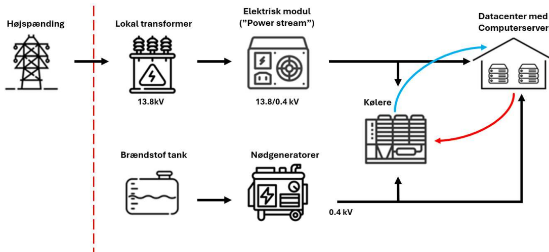
Figur 6: Princip for strømforsyning af datacentre. Stiplet rød linje er virksomhedens skel. De røde og blå linjer symboliserer varmt og afkølet vand.
