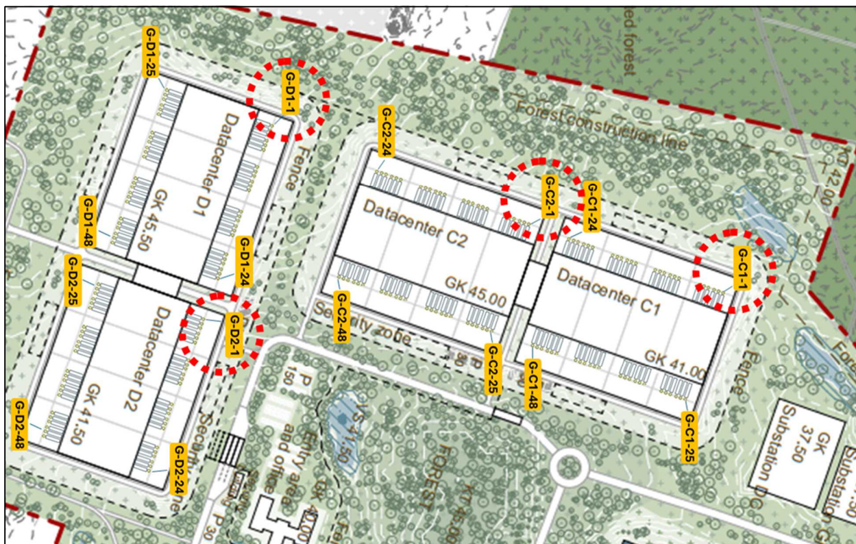
Figur 3-1 Illustration af placering af de fire afkast, som de fire generatorer der testes samtidigt men uafhængigt i beregningen, er tilsluttet.
