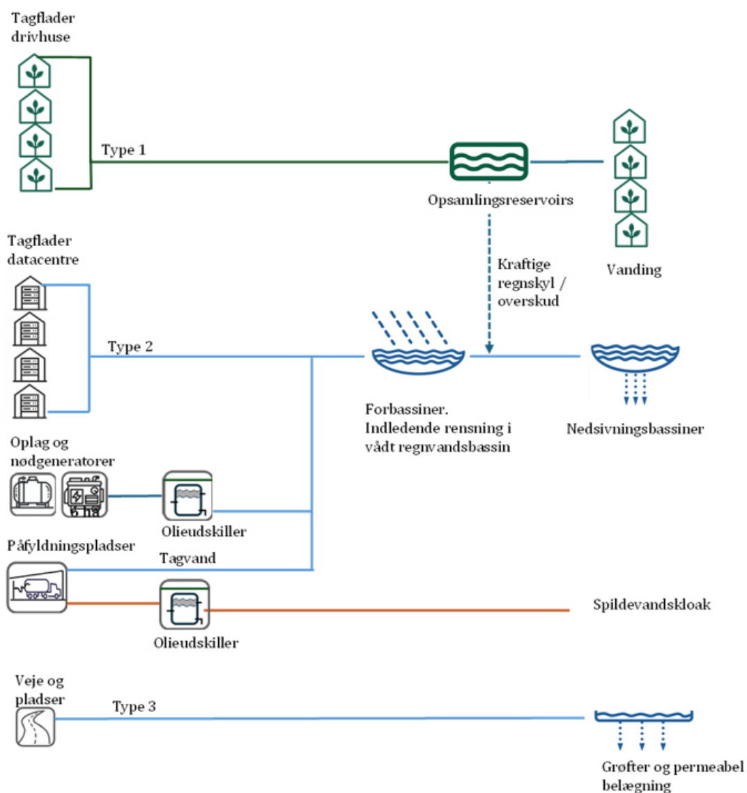
Figur 22: Principper for håndtering af regnvand
