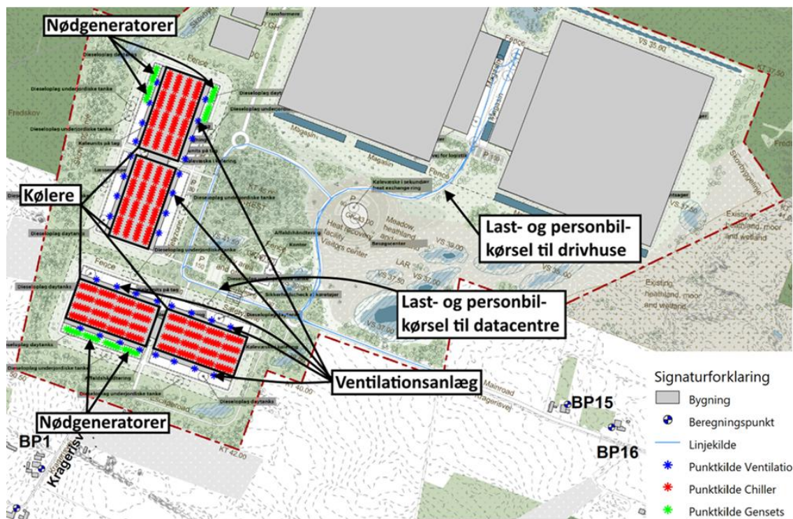
Figur 13: Placering af støjklender
