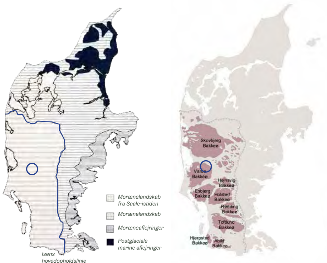
Figur 5.1 Isens hovedopholdslinje ved seneste istid (Weichsel)
