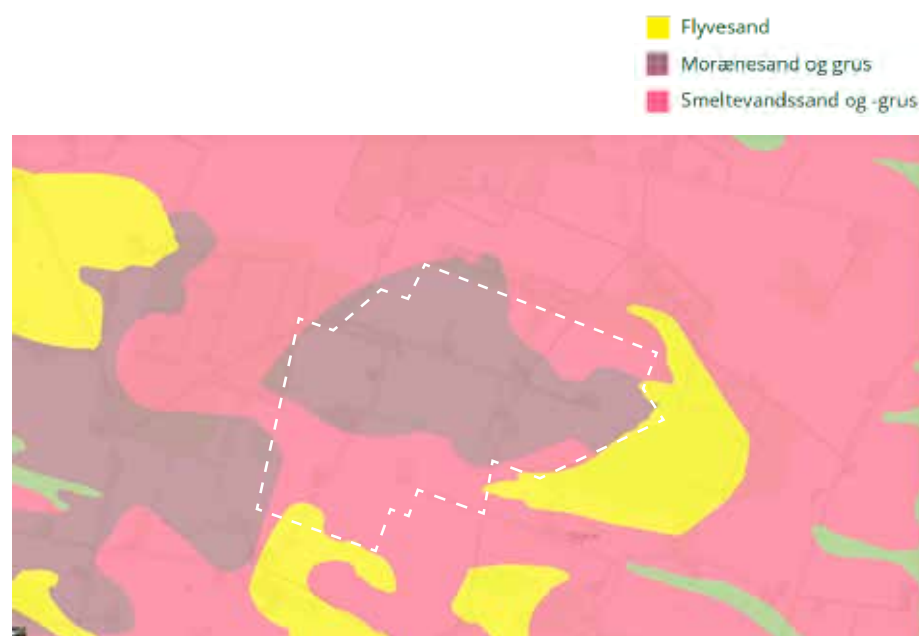
Figur 5.4 Jordartskort, GEUS, fra KAMP.klimatilpasning.dk
